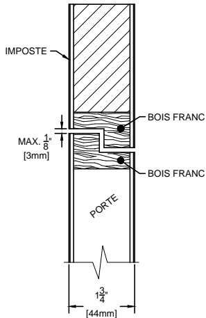
COUPE TRANSVERSALE DES TRAVERSES CONTIGÜES DE TYPE FEUILLURE
