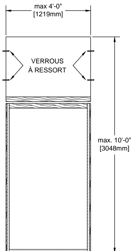
COUPE TRANSVERSALE DES TRAVERSES CONTIGÜES DE TYPE FEUILLURE
